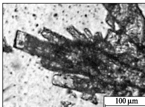
Рис. 4. Агрегат видовженопризматичних кристалів аланіту з прозорими головками, складеними епідотом Fig. 4. Aggregate of prismatic-elongated allanite crystals with transparent epidote tops
