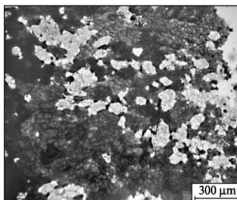
Рис. 5. Асоціація пізньої генерації аланіту (темний) з епідотом (світлий). Обидва мінерали з характерними тріщинами усушення Fig. 5. Association of later generation of allanite (dark) with epidote (light). Both minerals have characteristic shrinkage cracks
