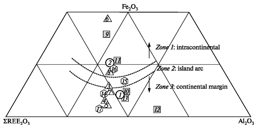
Рис. 6. Дискримінаційна діаграма Hoshino et al. [20] з фігуративними точками складу аланіту з геологічних комплексів УЩ. Нумери точок відповідають номерам аналізів у табл. 1
