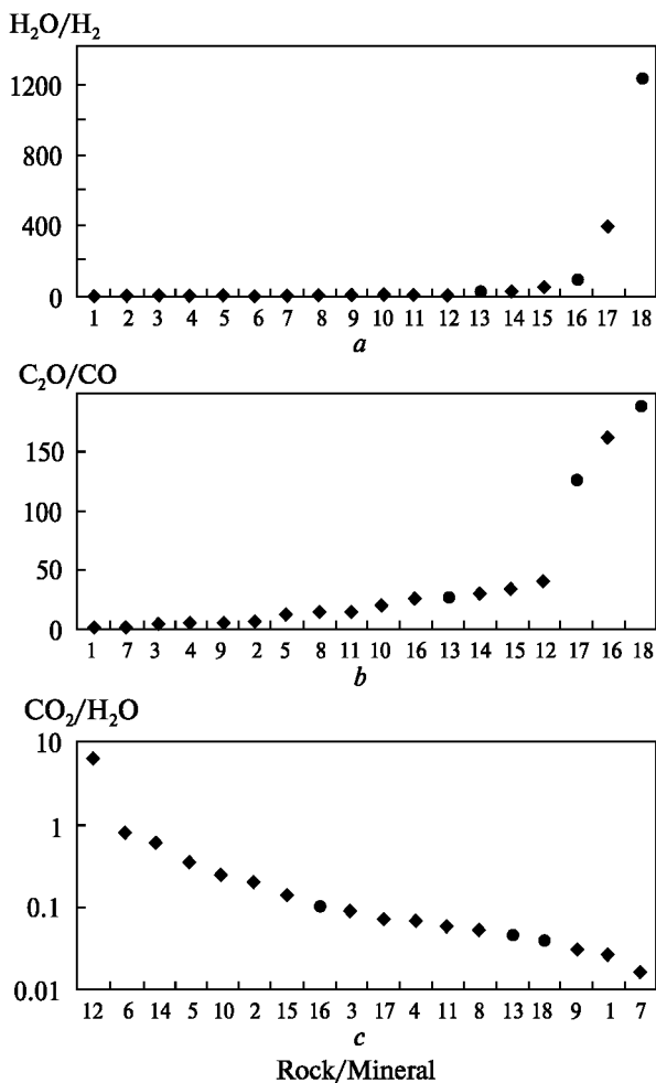
Рис. 8. Середні співвідношення молекулярної кількості H_2O/H_2 , CO_2/CO і CO_2/H_2O у продуктах піролізу (250–1050 °C) порід і мінералів деяких геологічних об'єктів УЩ (у дужках зазначено кількість аналізів): 1 — граніт новоукраїнський (2); 2 — пегматити Коростенського плутону (18); 3 — пегматити Корсунь-Новомиргородського плутону (6); 4 — граніт анадольський (3); 5 — сієніти Азовського штоку (49); 6 — сієніти Яструбецького масиву (29); 7 — пегматити Полохівського поля (30); 8 — граніт салтичанський (2); 9 — граніт стародубовський (2); 10 — породи Октябрського масиву (19); 11 — пегматити Шевченківської тектонічної зони (9); 12 — породи Чернігівського масиву (30); 13 — аланіт салтичанського граніту; 14 — сієніти Покрово-Київського масиву (12); 15 — граніт хлібодарівський (3); 16 — аланіт-1 Анадольського рудопрояву; 17 — жильна порода цього рудопрояву; 18 — аланіт-2 цього рудопрояву
